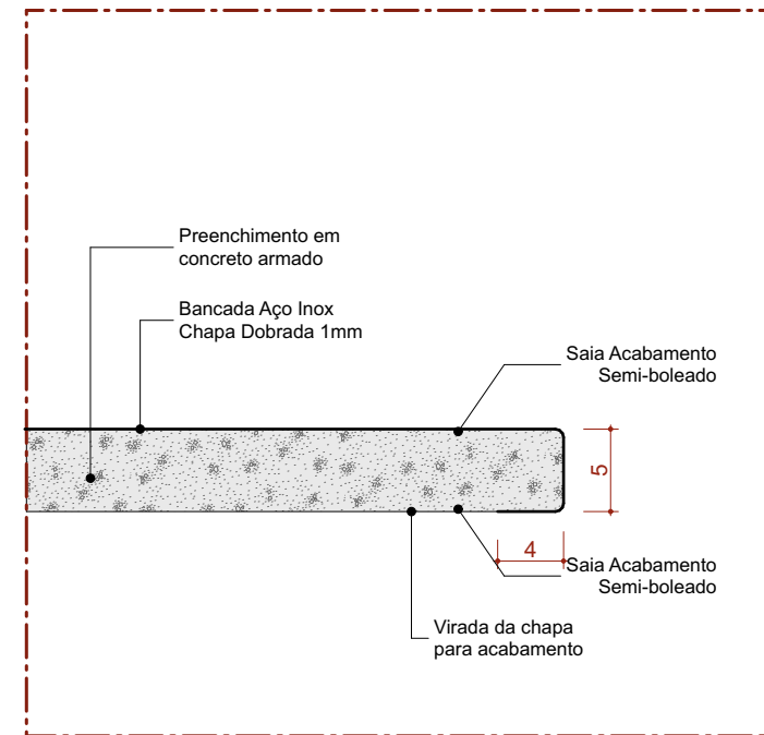
Det. B.I.d Bancada de Inox Detalhe Saia - Área seca
