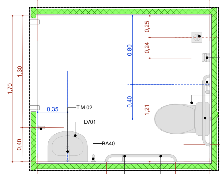
A.M.2 Sanitário PCD Fem. Escala:1:25
