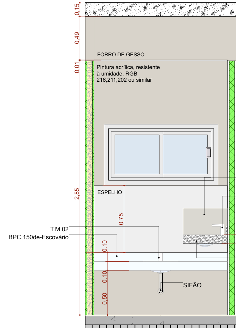
A.M.04 VISTA 2 Escala:1:25
