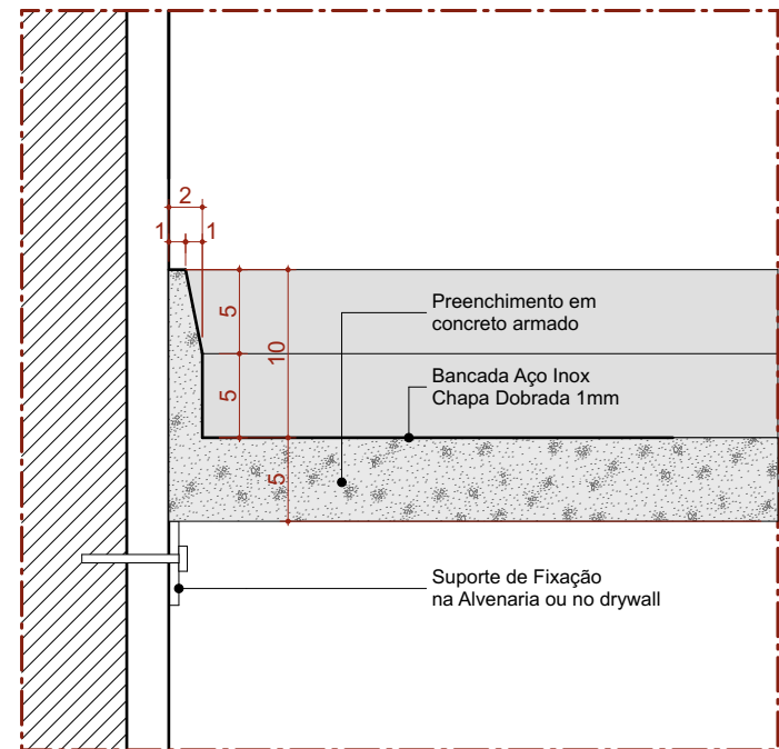
Det. B.I.c Bancada de Inox Detalhe Frontão - Área Seca
